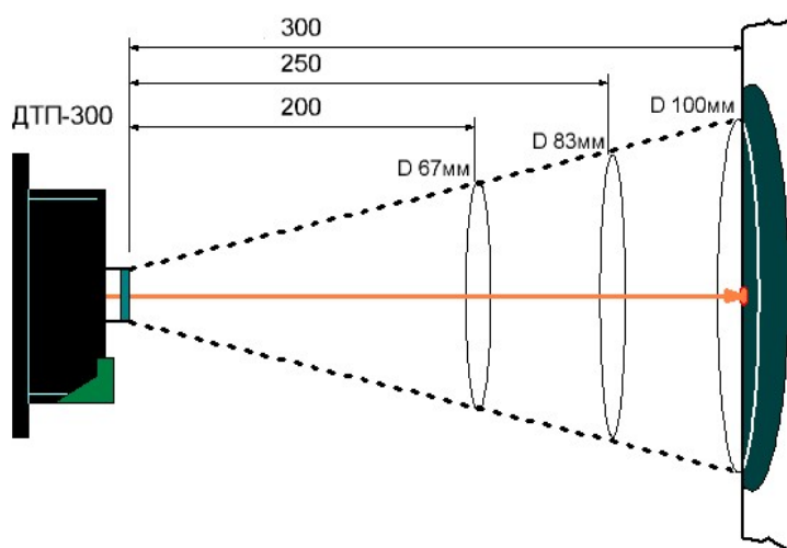
Рисунок №5. Расположение датчика ДТП-300 с оптическим соотношением 3:1.
